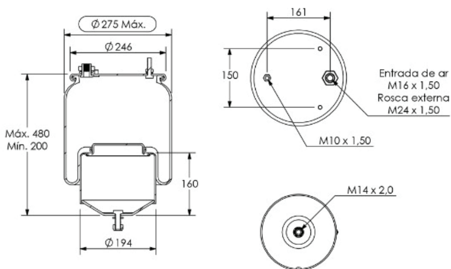
CAMARA DE AIRE TUBULAR (ST230) VOLVO FH / FM 2015 EN ADELANTE (4560N) TAPA CON NIPLE DE 3/4 Y SUJECION
